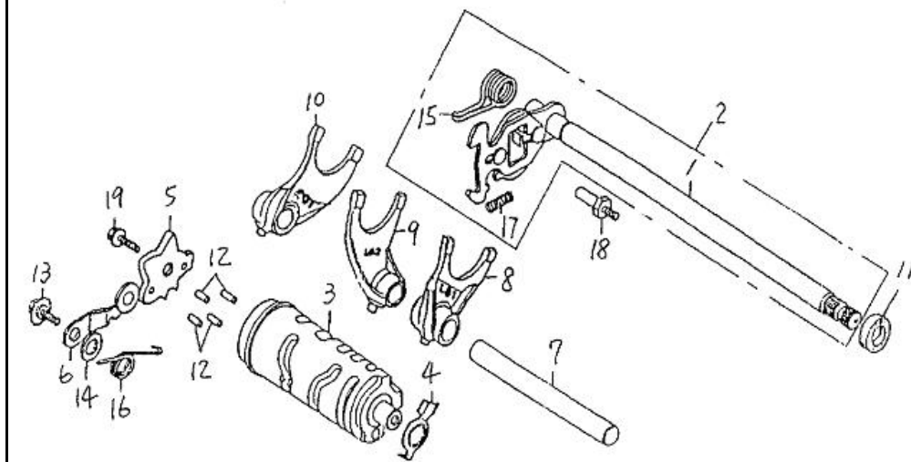
FIG 12 GEAR SHIFT
