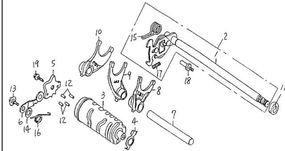
FIG 12 GEAR SHIFT
