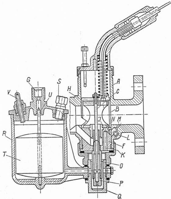
Bild 16. Vergaser R 51 (R 61 und 66)
