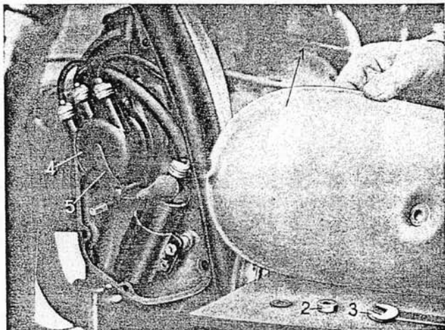
Bild 8. Zündanlage R 61 (R 66—71)
