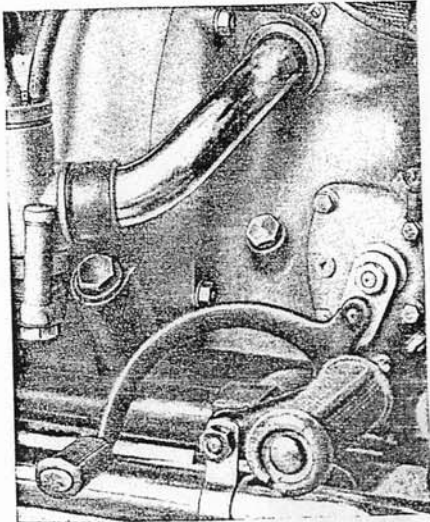
Bild 20. Fußschalthebel
