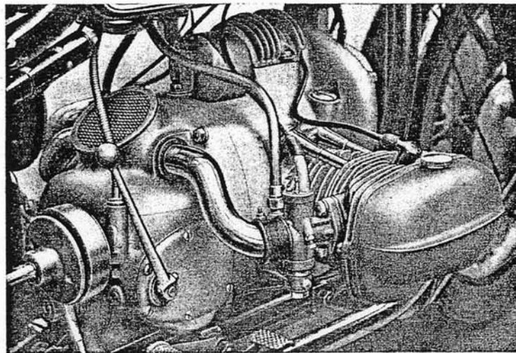
Bild 13. Motorblock R 51
