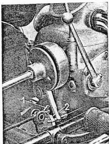
Bild 12. Brems- und Kupplungsnachstellung
