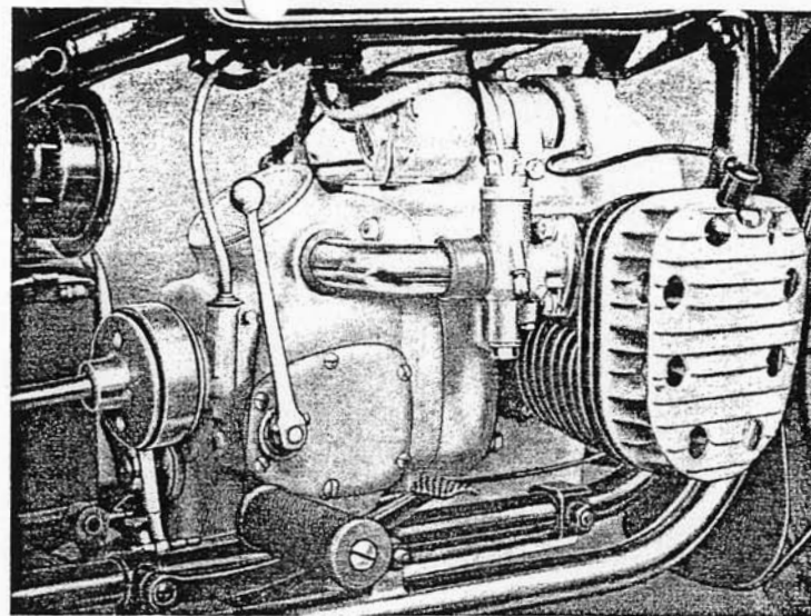
Bild 5. Motoranlage R 71
