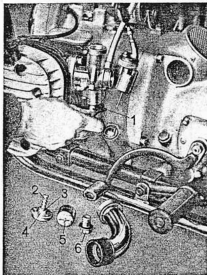
Bild 4. Vergaser R 71
