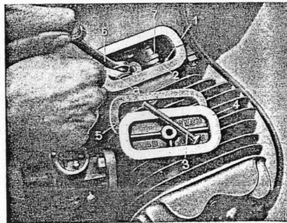
Bild 7. Ventilaachstellung R 61 (R 71)
