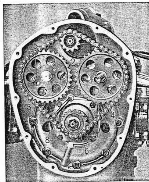
Bild 14. Stirnräderantrieb R51
