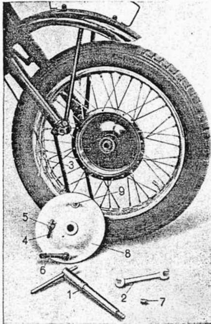
Bild 1. Ausbau des Vorderrades
