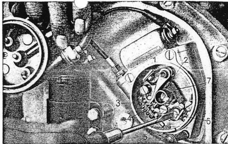
Bild 9. Unterbrecher
