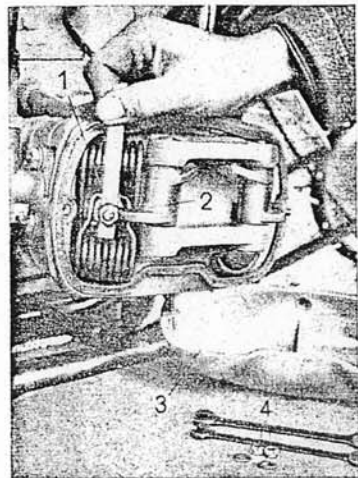
Bild 6. Zylinderkopf R 66 (R 51)
