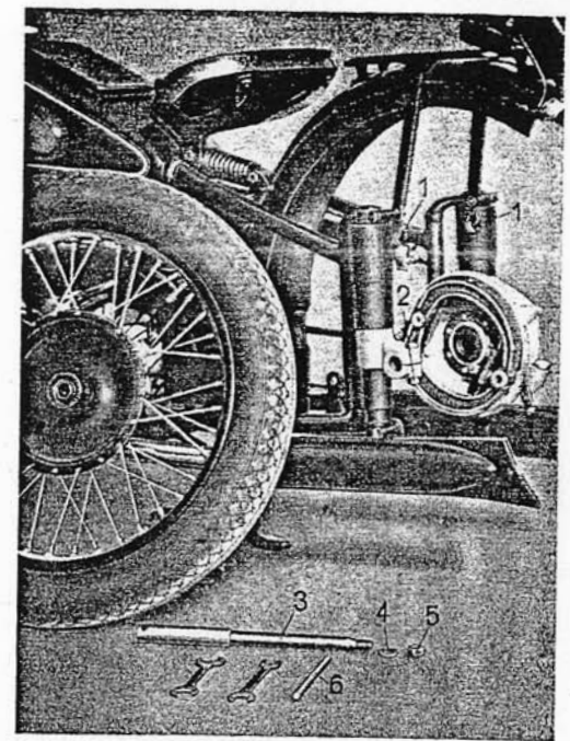
Bild 2 Ausbau des Hinterrades
