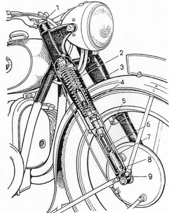
Bild 21. Vorderradgabel
