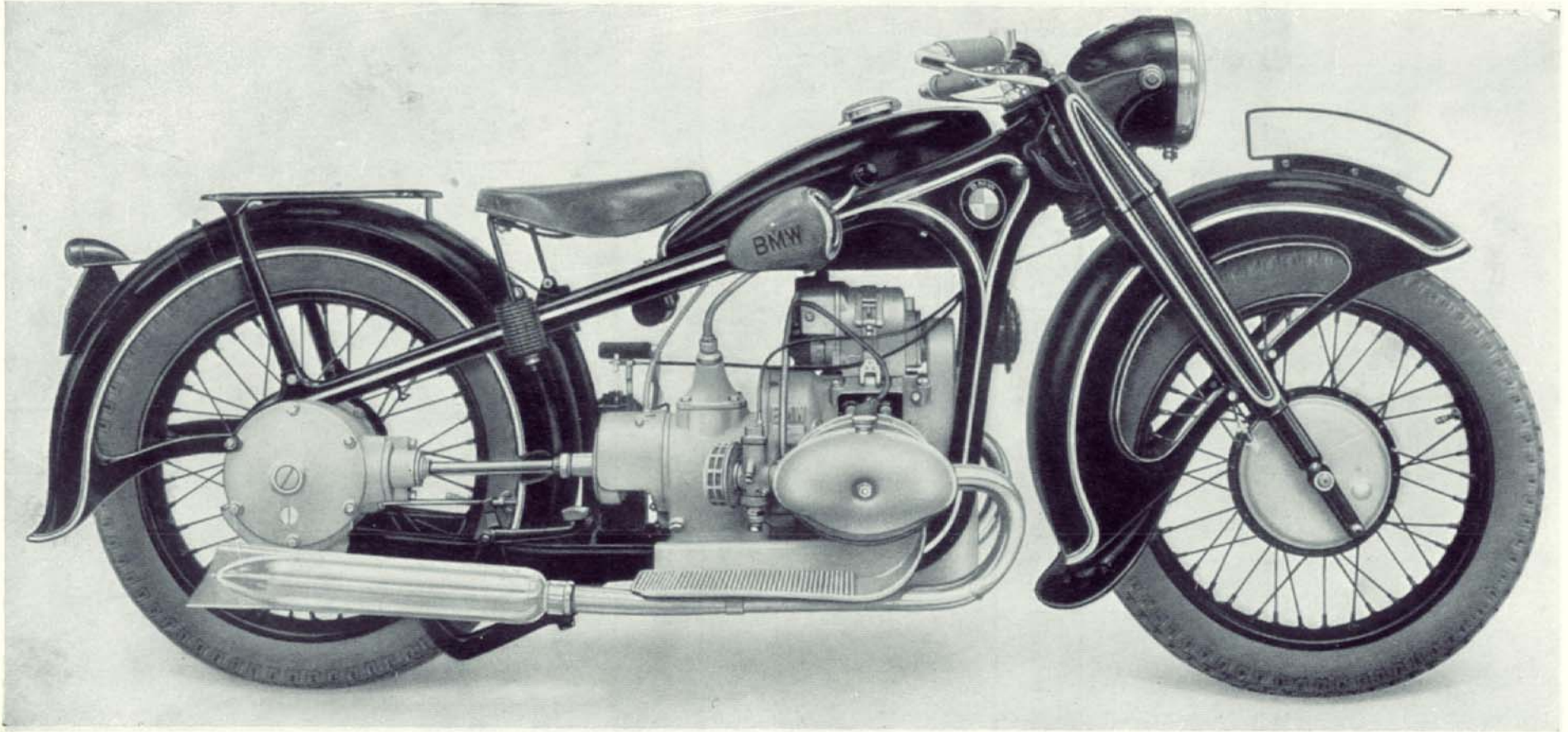
R 17-Maschine von der Antriebsseite aus
