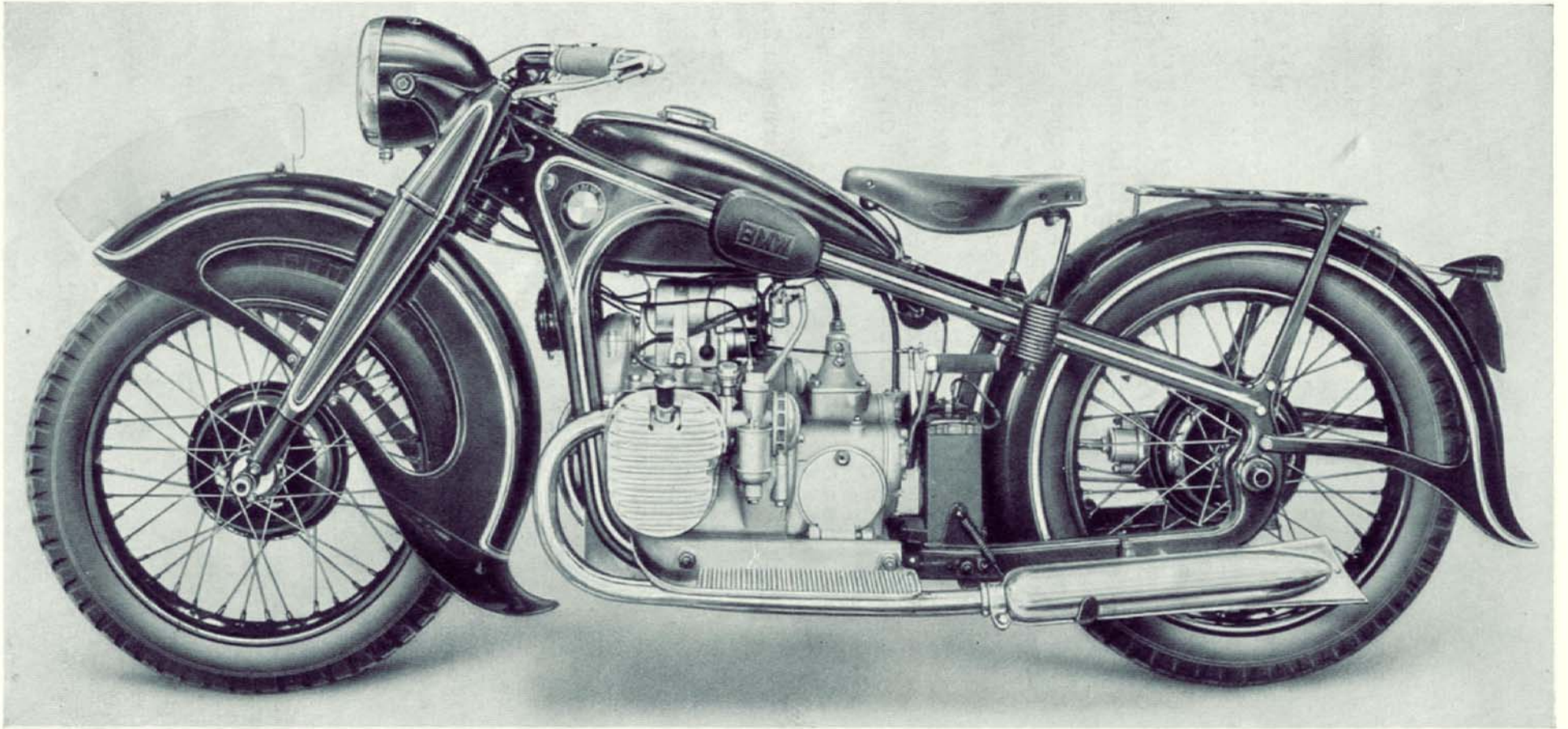
R 12-Maschine von der Fußanwerfhebelseite aus
